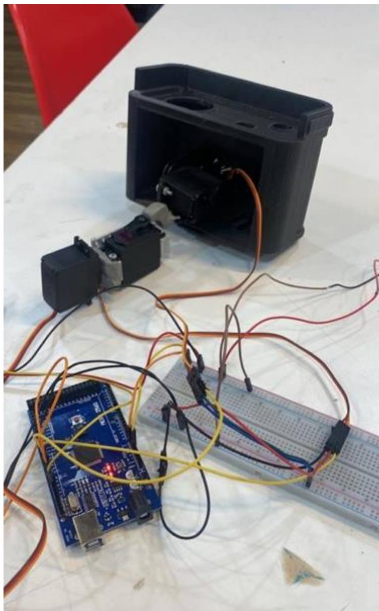
Figura 1 Droid em construção
